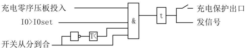
充电零序逻辑图
