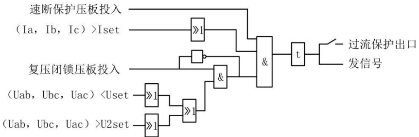
过流保护逻辑图
