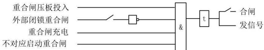
重合闸逻辑图
