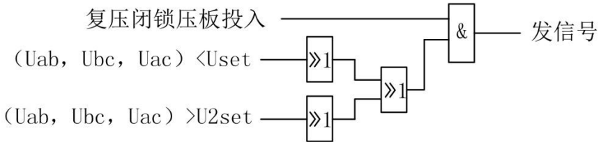
复压闭锁逻辑图
