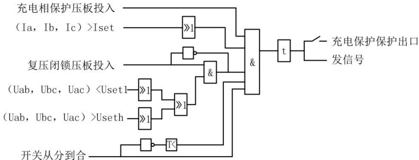
充电保护逻辑图
